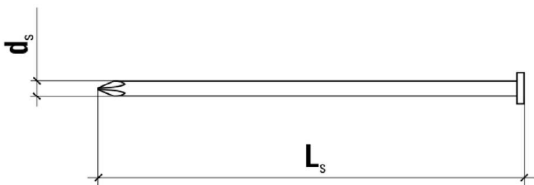
Spezialnagel TGX-4,4
