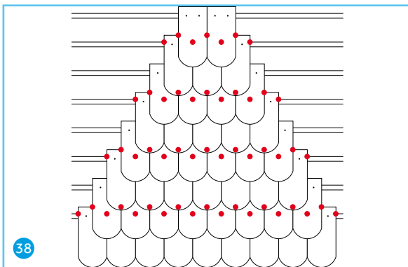
Opal Doppeldeckung mit Opal Sturmklammer Plus, 2:1 jede 2te Reihe
