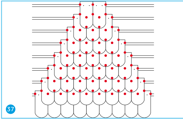
Opal Doppeldeckung mit Opal Sturmklammer Plus, 2:1 jede Reihe
