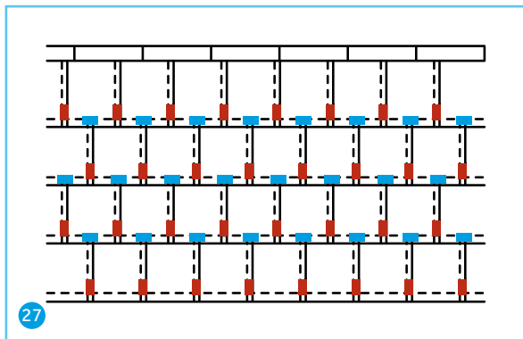
Tegalit Aerlox mit Braas Clip (Rot) und Kopf-/Falzklammer (Blau), 2x (1:1)
