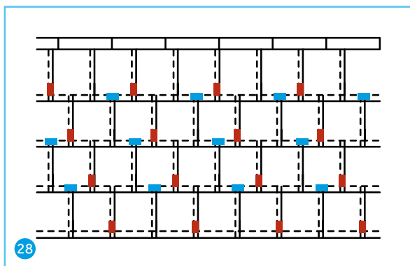
Tegalit Aerlox mit Braas Clip (Rot) und Kopf-/Falzklammer (Blau), 2x (1:2)
