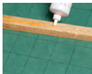
2. Divoroll Dichtmasse auf die Konterlatte auftragen
